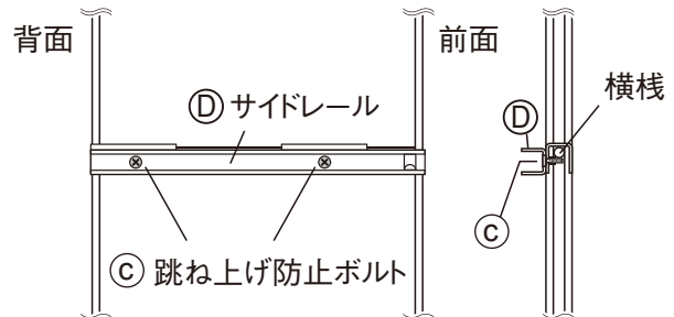
跳ね上げ防止ボルト取り付け位置
