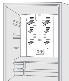
冷蔵庫冷気吹出口図
