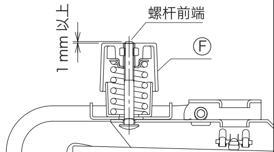
图 1 拧紧手柄的参考
