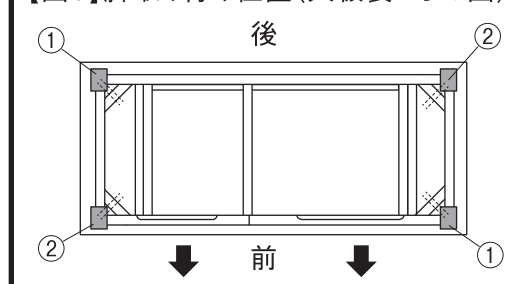
【図1】脚取り付け位置(天板裏からの図)
