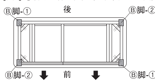
【図1】⑥脚取り付け位置（天板裏からの図）
