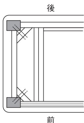
【図2】 ⑥脚取り付け位置の説明
